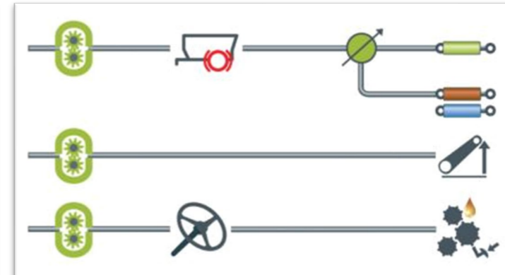
TRE HYDRAULIKKUMPER
